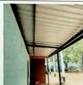
Foto 5: MODULO B Vista exterior Corredor. Se sustituyo la cubierta de lamina de zinc por lamina troquelada cal 26. Se le dio mantenimiento a las costaneras de metal.
