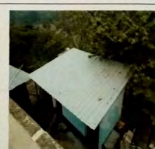
Foto 6: MODULO D Sustitucion de cubierta de lamina de zinc por lamina troquelada cal 26.
