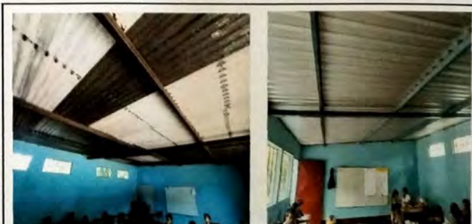
Foto 18: MODULO AULA A LA PAR DE MODULO DE PRE PRIMARIA. Vista Interior Se le dio mantenimiento a y estructura de metal y se sustituyo la lamina de zinc por lamina troquelada cal 26.
